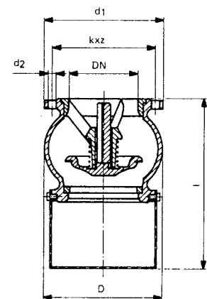
Baureihe 302, DN 125-150
